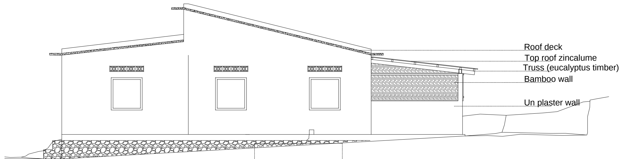
RIGHT ELEVATION
