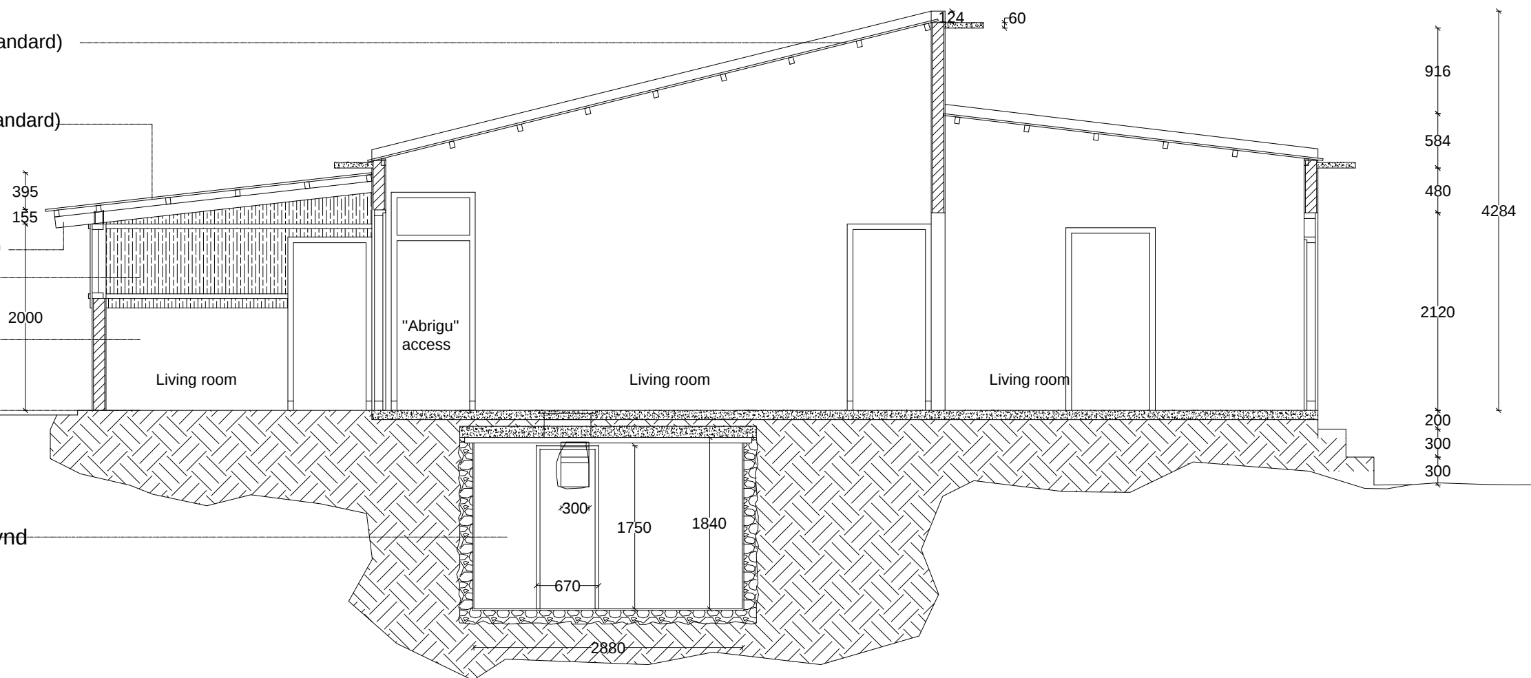
SECTION A-A 1:200
