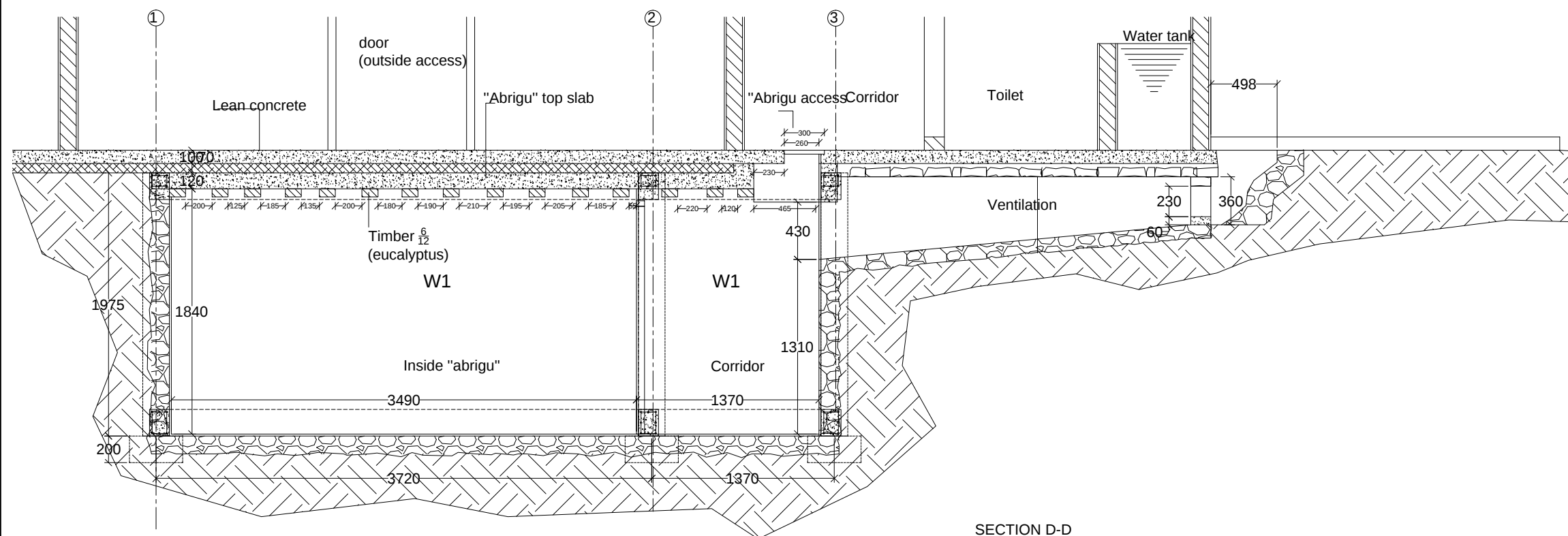
SECTION D-D
