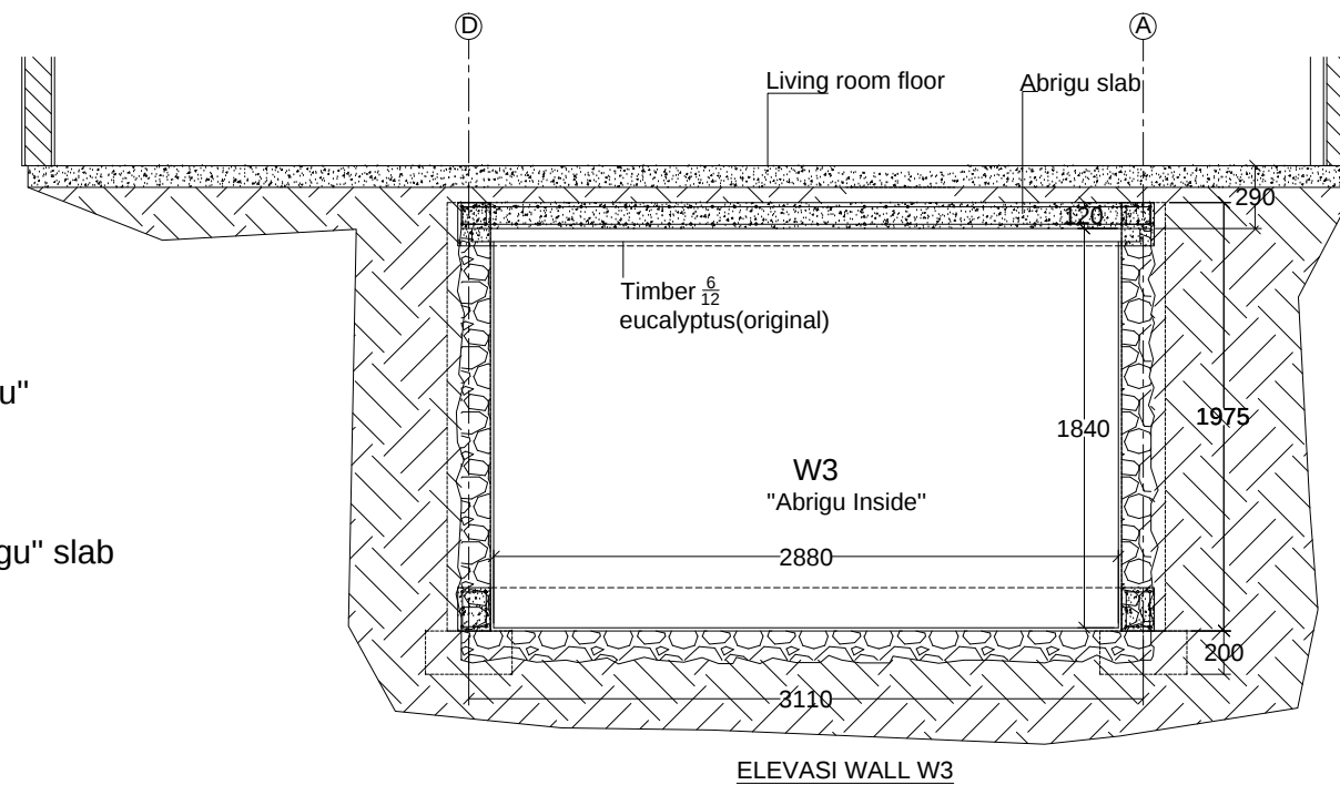
"ABRIGO" ELEVATION 1:200
