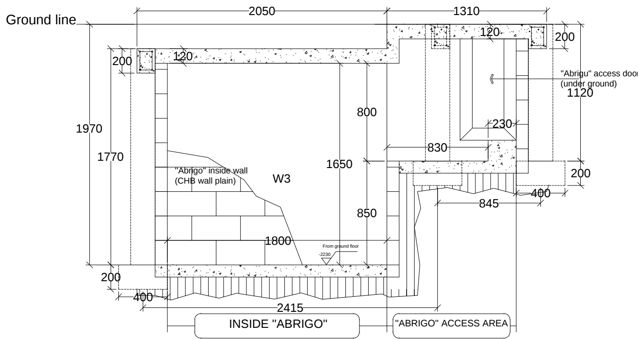
"ABRIGU SECTION F1-F'1 1:1000
