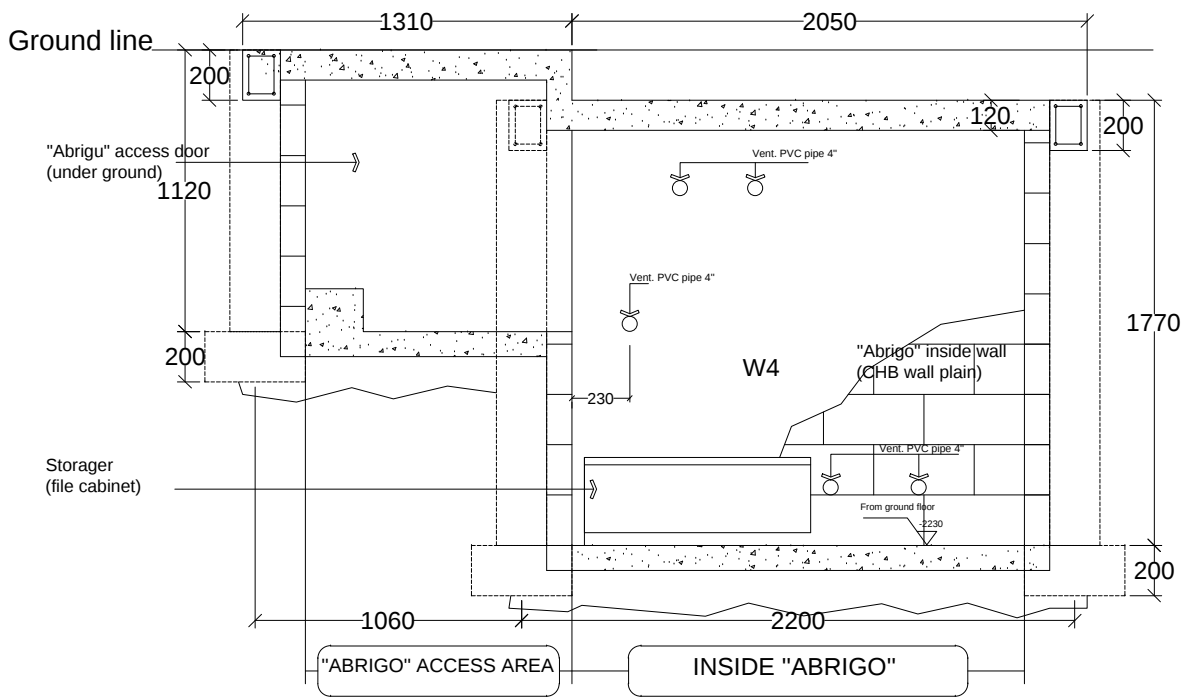
"ABRIGU SECTION G1-G'1 1:1000
