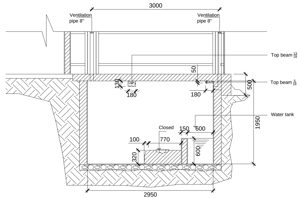
SECTION D-D
